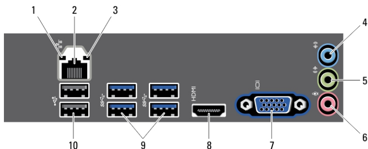
איור 2. תצוגת לוח אחורי
